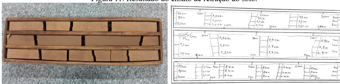
Figura 11: Resultado do ensaio de retração do solo.
